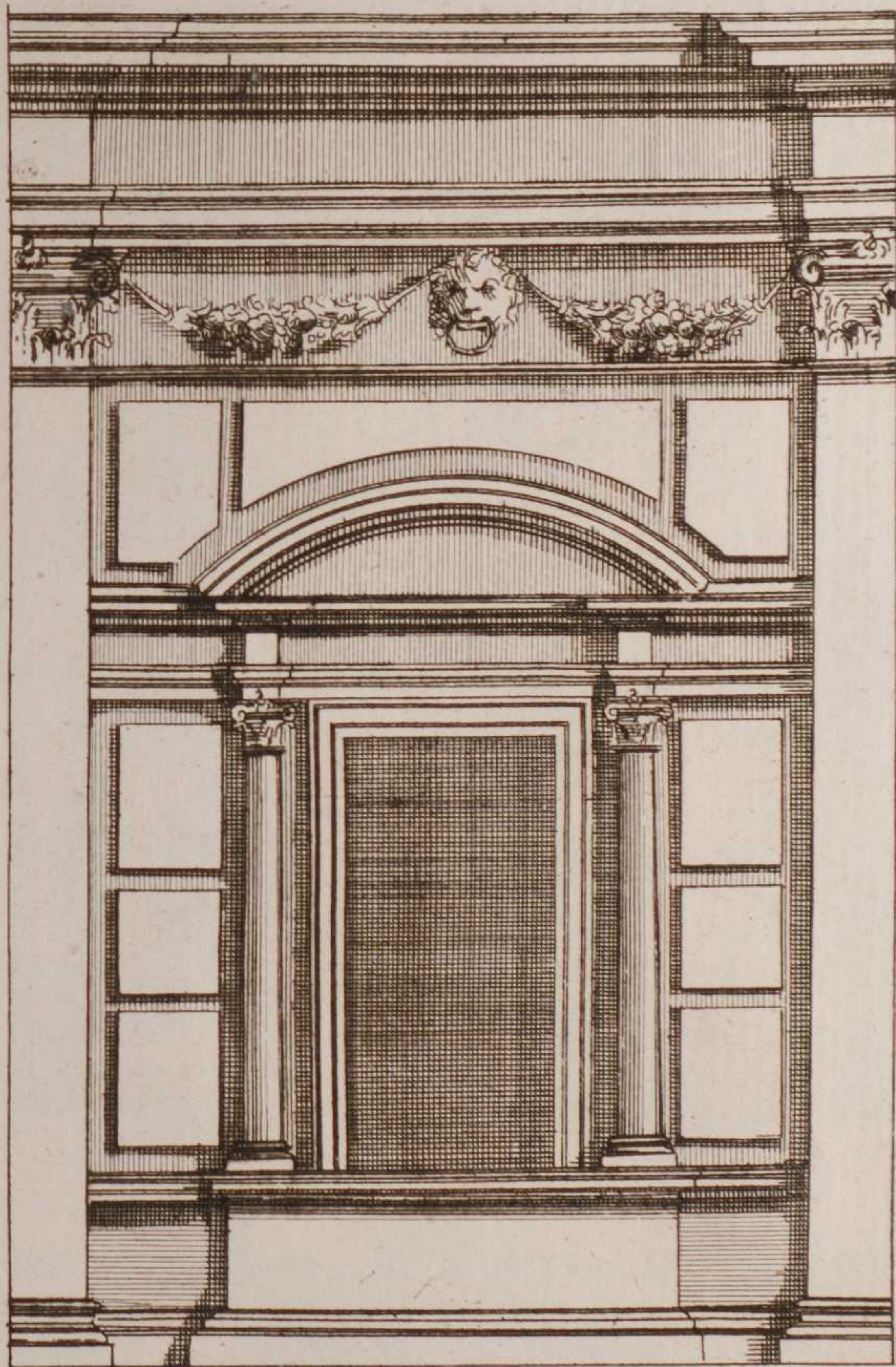
Arch: di Andrea Palladio
